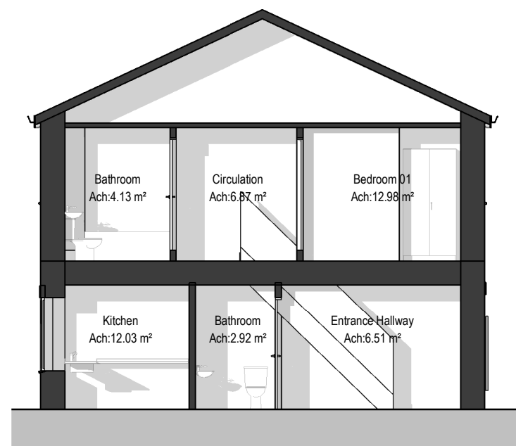
H2 Section B 1 : 100
