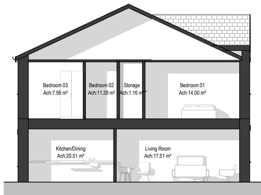
SSA H3 Section B 1 : 100
