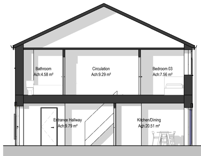
SSA H3 Section A 1 : 100
