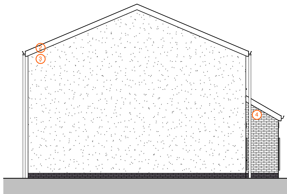
F2.2 Side Elevation 033 1 : 100
