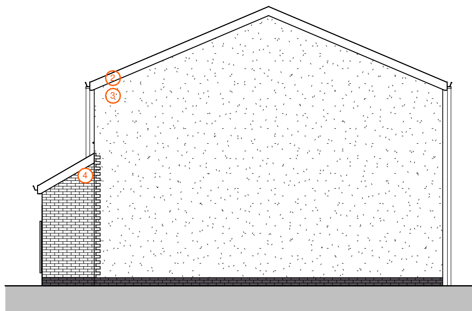
F2.2 Side Elevation 044 1 : 100
