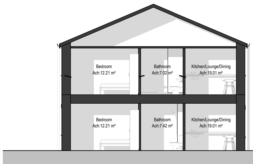
F2.2 Section A 1 : 100
