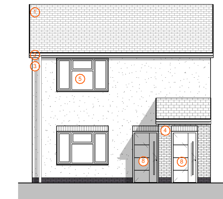
F2.2 Front Elevation 01 1 : 100
