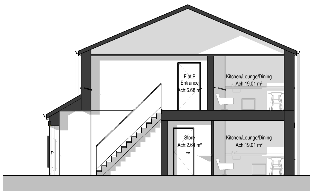
F2.2 Section B 1 : 100
