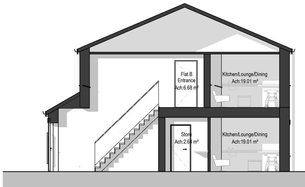
F2.1 Section B 1 : 100
