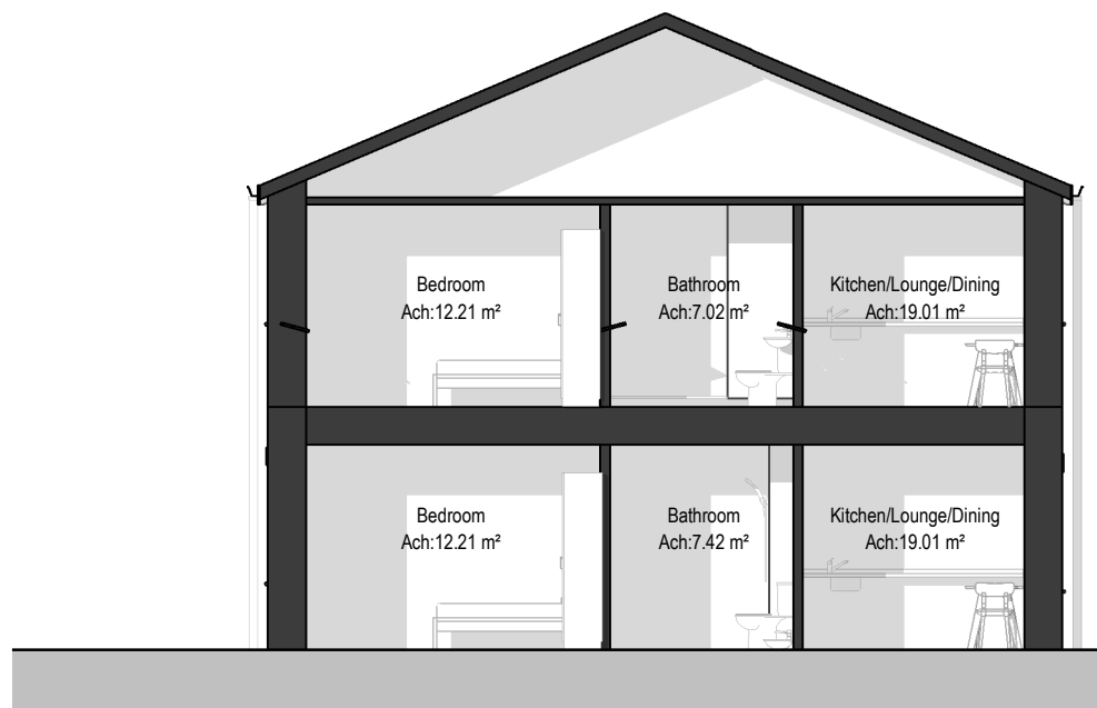
F2.1 Section A 1 : 100
