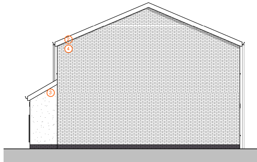
F2.1 Side Elevation 04 1 : 100
