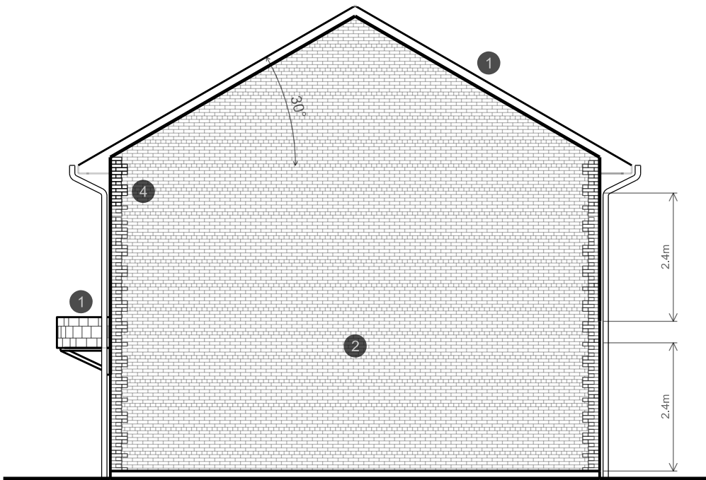
Type H3 - 5P2B Right Elevation
