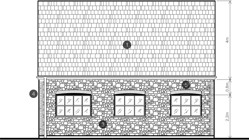
Type B1 - 3P2B - Bungalow Back Elevation
