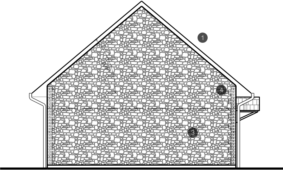
Type B1 - 3P2B - Bungalow Left Elevation
