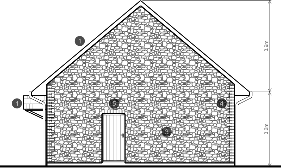
Type B1 - 3P2B - Bungalow Right Elevation
