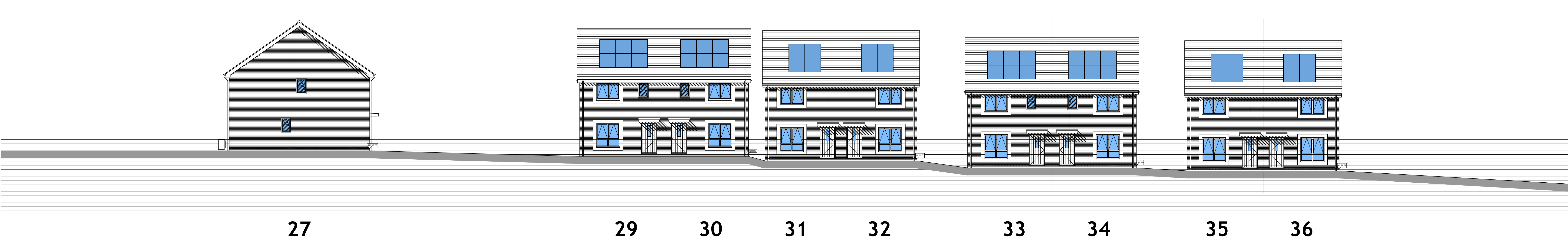
2.6.2.D Site Section D-D / Adran Safle D-D
