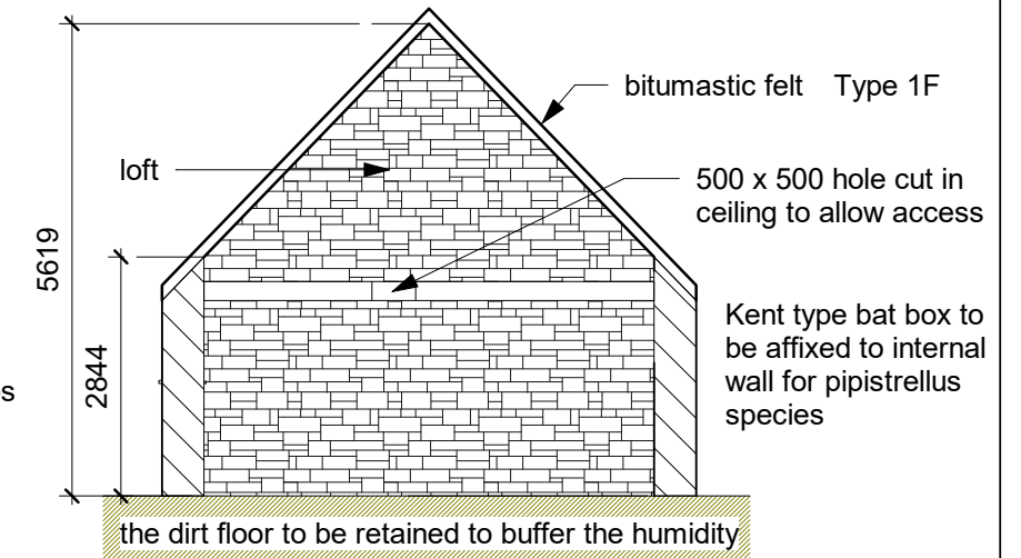
6 Section 1 1 : 100
