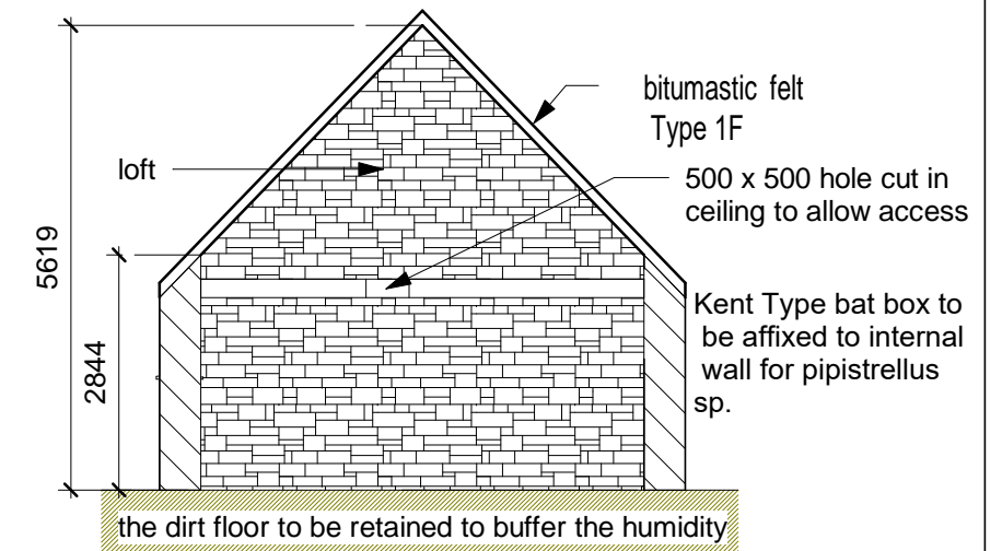
6 Section 1 1 : 100
